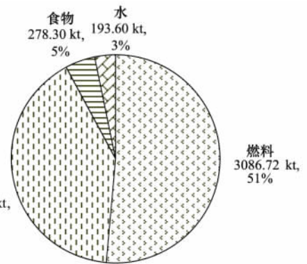
图 6 厦门市 2009 年城市主要材料内含能碳足迹 (CO 2 e)
