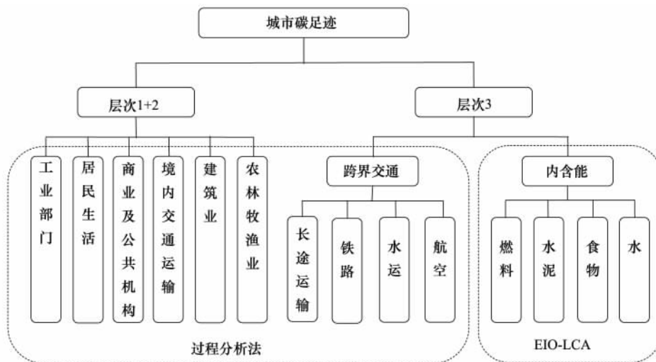
图1 城市碳足迹混合分析方法
