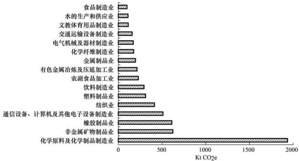
图 4 厦门市 2009 年工业部门中行业的碳足迹
