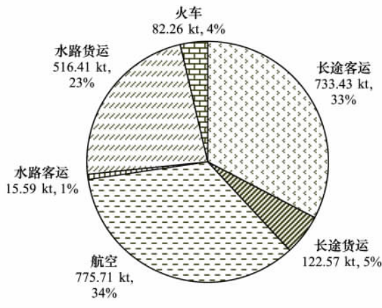
图 5 厦门市 2009 年跨界交通碳足迹 (CO 2 e)
